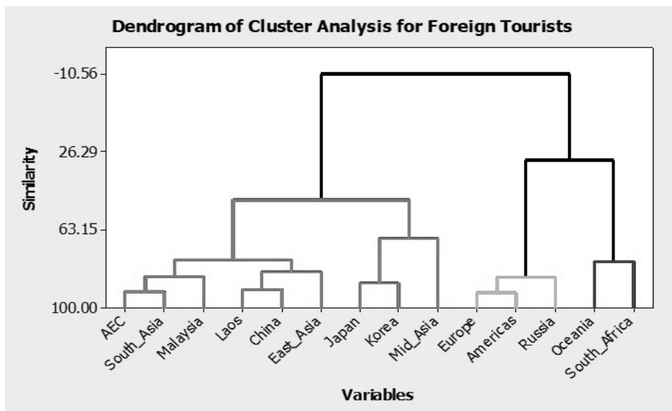
ภาพที่ 1 เดนโดแกรมของการวิเคราะห์การแบ่งกลุ่มสำหรับนักท่องเที่ยวชาวต่างชาติ
